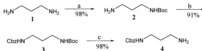
Scheme 4. (a) (\text{Boc})_2\text{O/CHCl}_3/0^\circ\text{C} ; (b) \text{CbzCl/THF/NaOH(3.3 N)} ; (c) \text{TFA/CH}_2\text{Cl}_2 .
